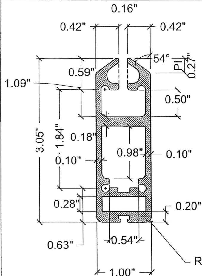
(4B) BOTTOM BAR 6063-T6 ALUM. ALLOY
